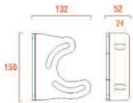
Universalträger
