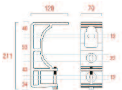
Universalträger
