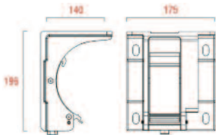
Universalträger
