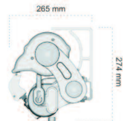
Neigung 60°
