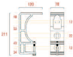
Universalträger
