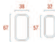
Querschnitt Armprofil
